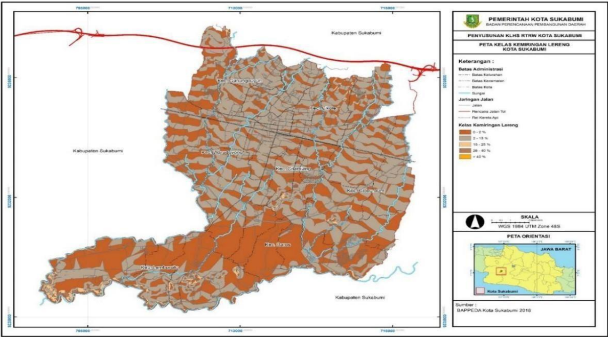
Gambar 2.4 Peta Kemiringan Lereng Kota Sukabumi
