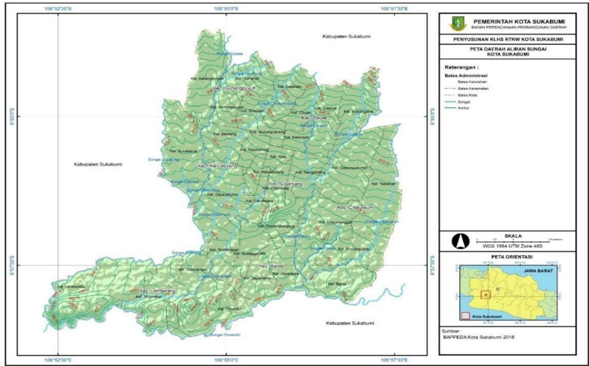
Gambar 2.7 Peta Daerah Aliran Sungai di Kota Sukabumi
