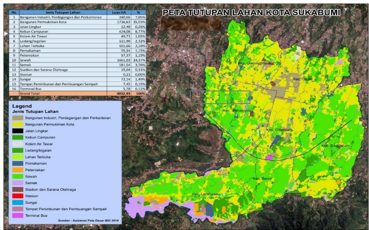
Gambar 2.8 Peta Tutupan Lahan Kota Sukabumi
