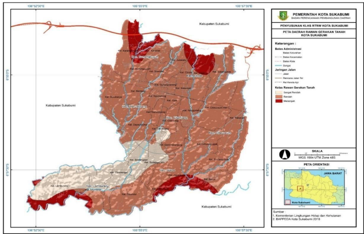
Gambar 2.5 Peta Rawan Gerakan Tanah di Kota Sukabumi
