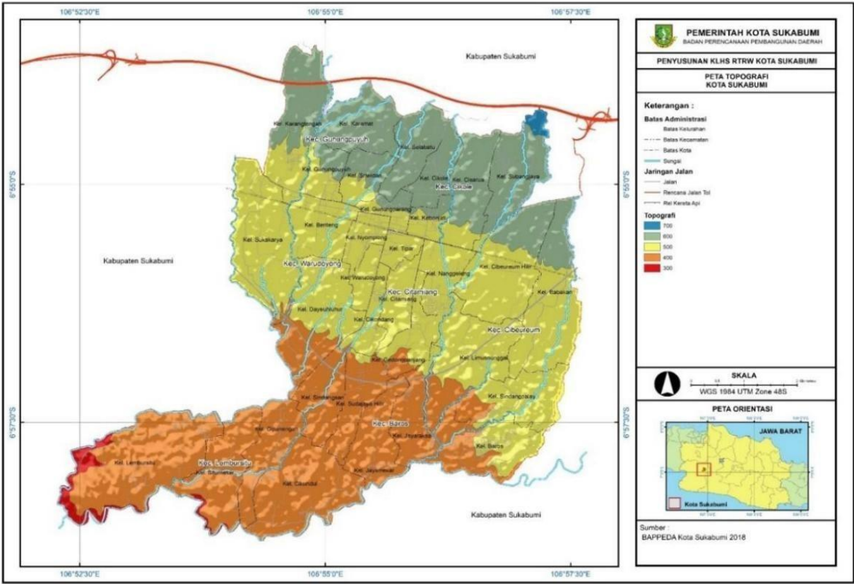
Gambar 2.3 Peta Topografi Kota Sukabumi
